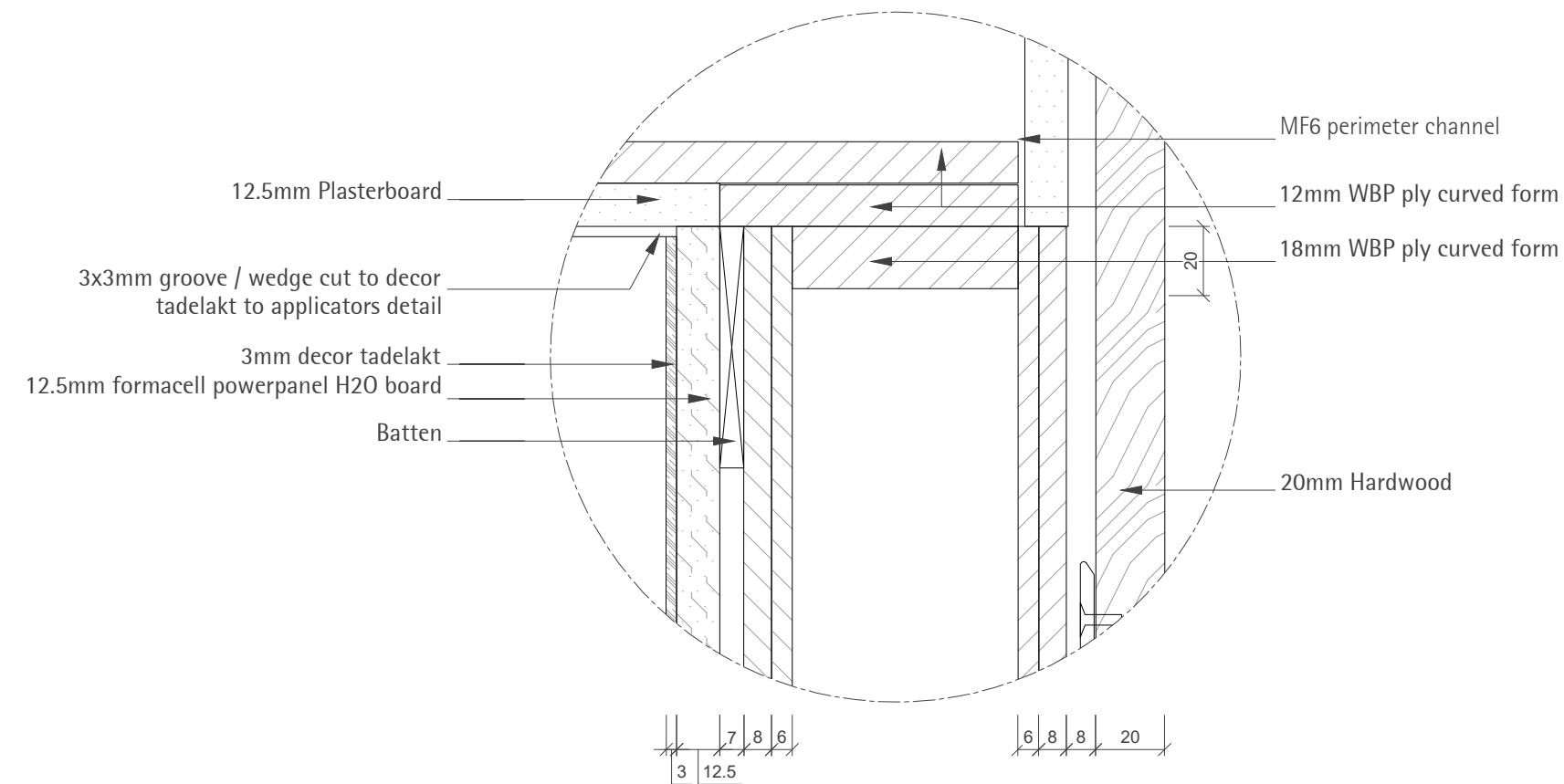
DT05 DETAIL SCALE 1:2
