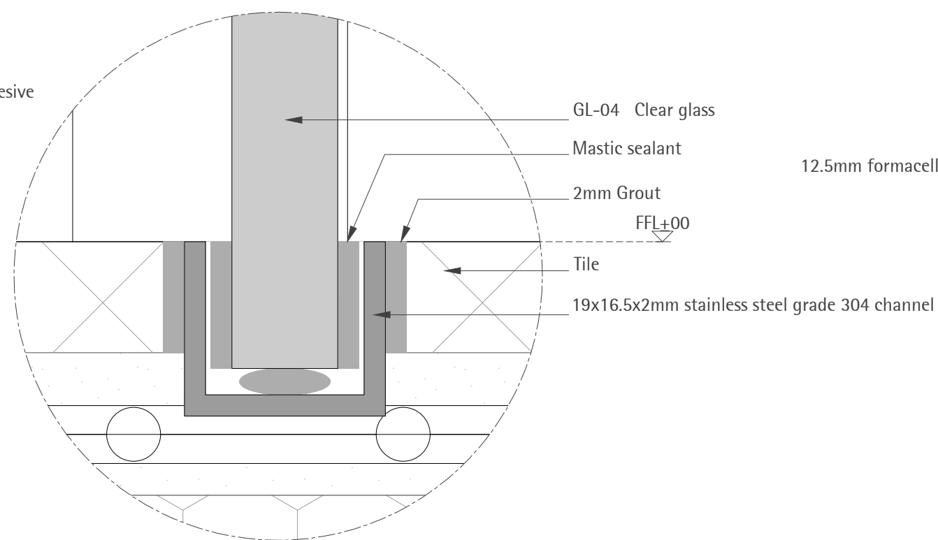
DT04 DETAIL SCALE 2:1
