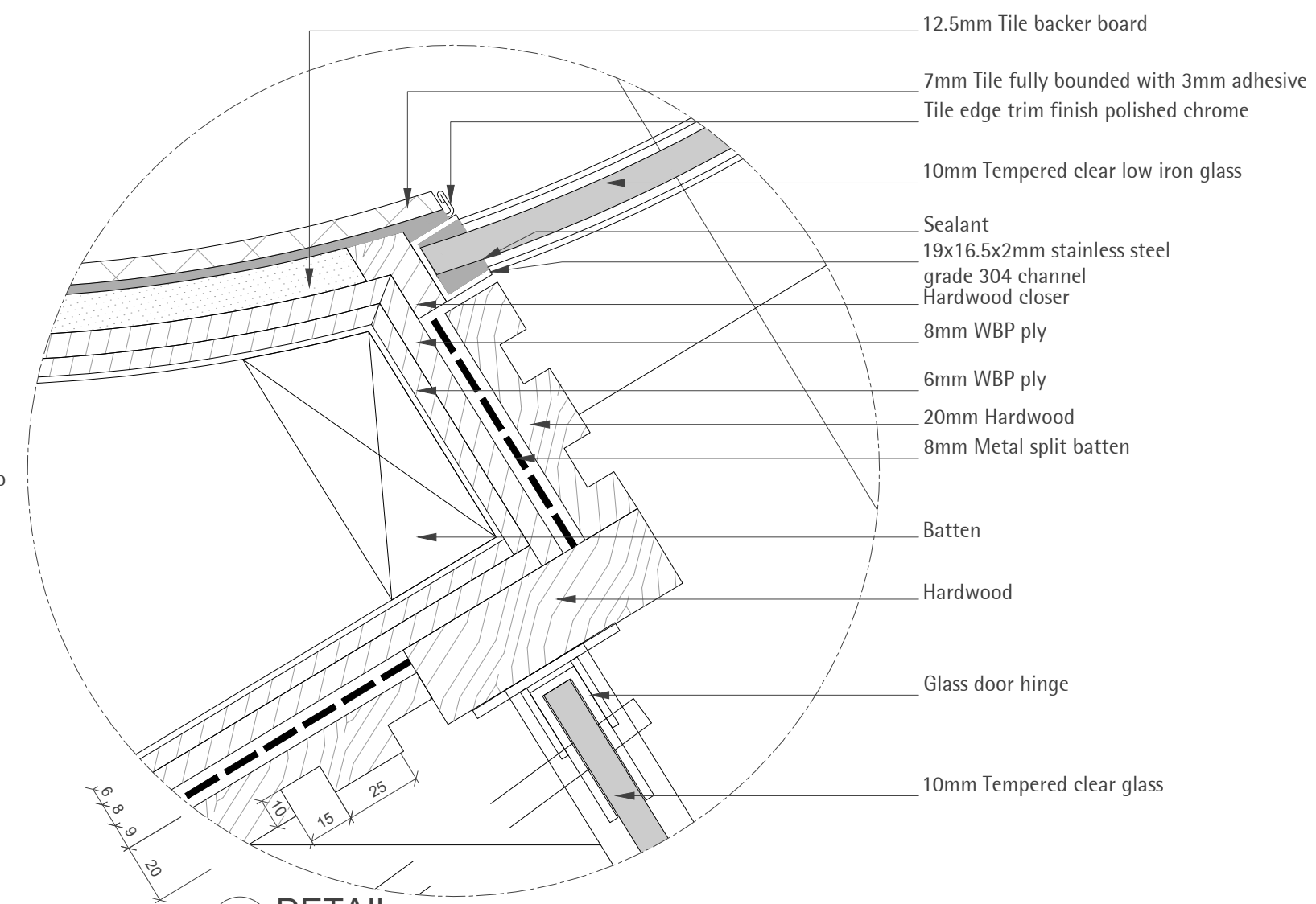
DT05 DETAIL SCALE 1:2
